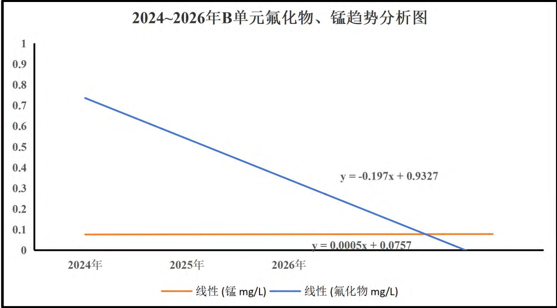
图 8.2-4 2024~2026 年 B 单元氟化物、锰趋势分析图
