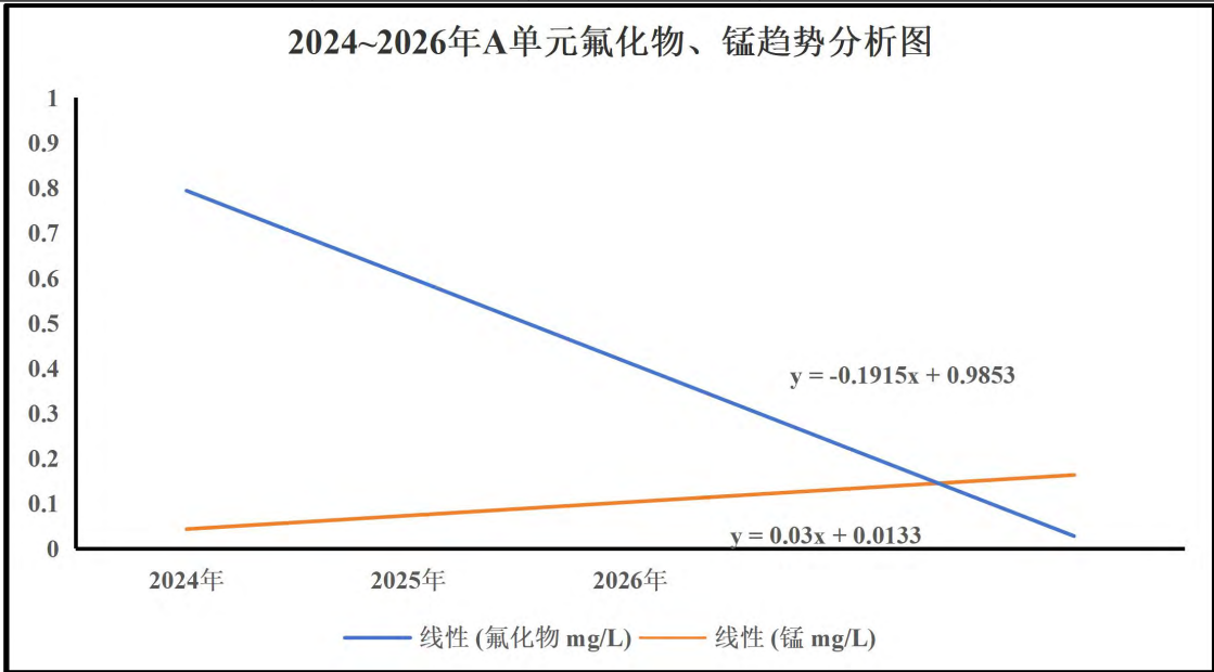
图 8.2-1 2024~2026 年 A 单元氟化物、锰趋势分析图
