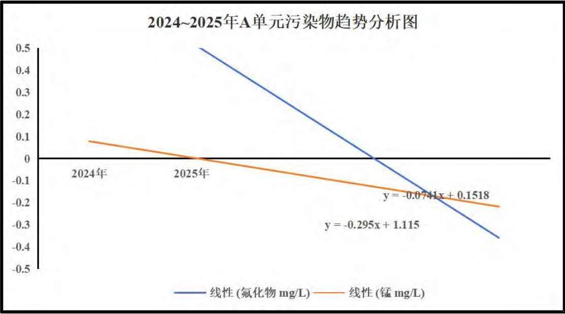
图 2.3-7 2024~2025 年 A 单元污染物趋势分析图
