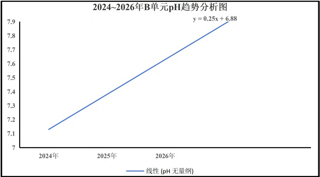
图 8.2-5 2024~2026 年 B 单元 pH 趋势分析图
