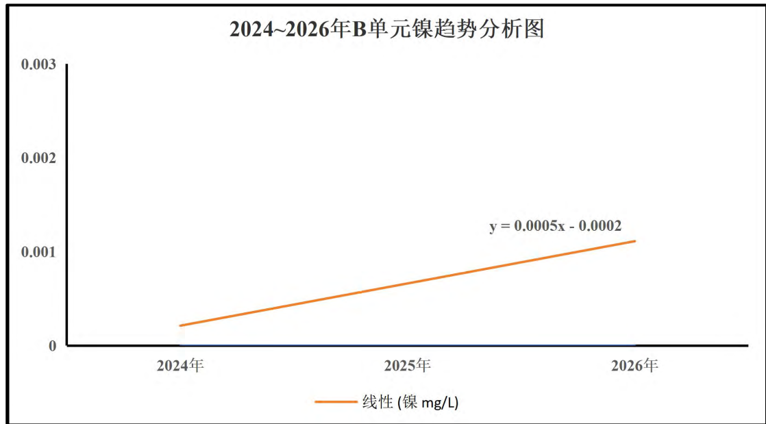
图 8.2-6 2024~2026 年 B 单元镍趋势分析图
